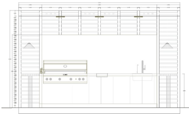
Plano de arquitectura de la zona de quincho.
